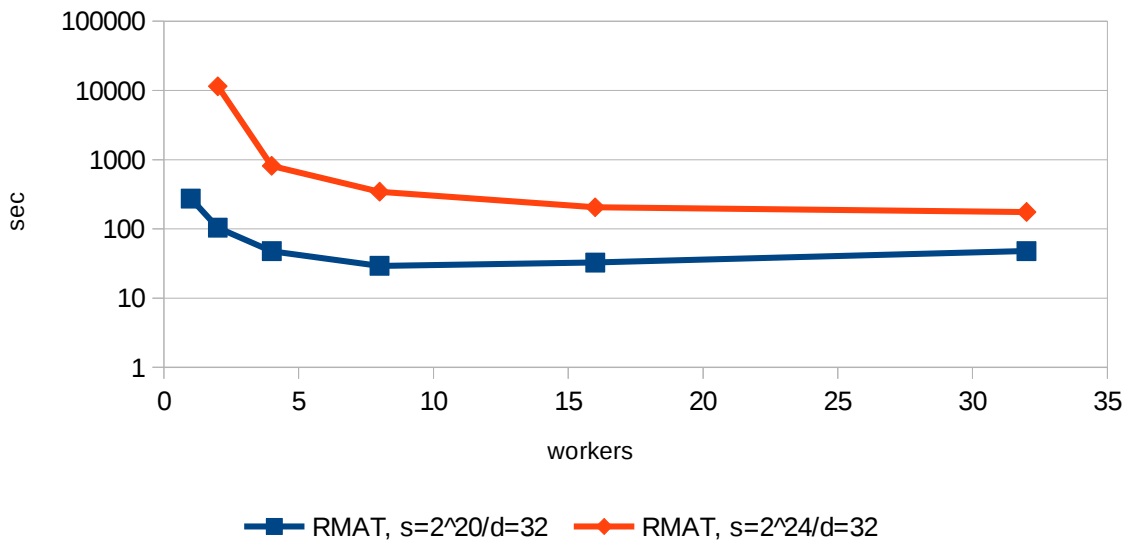
Fig. 1. Scalability (y — log scale).
